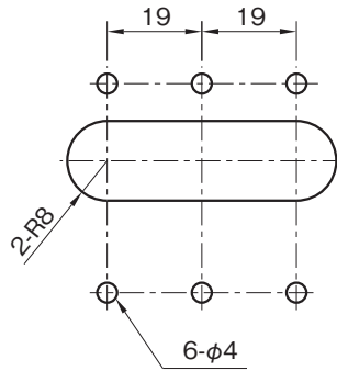
取付穴加工図 (公差:±0.1)
