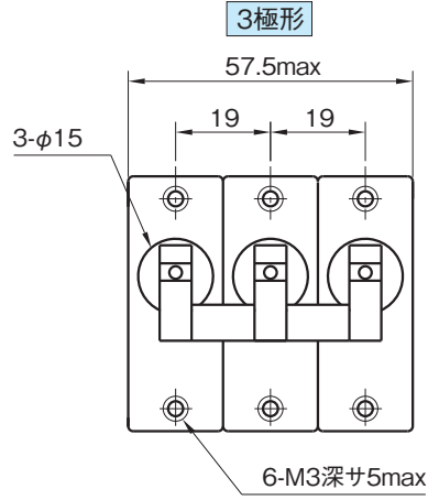
取付穴加工図 (公差:±0.1)
