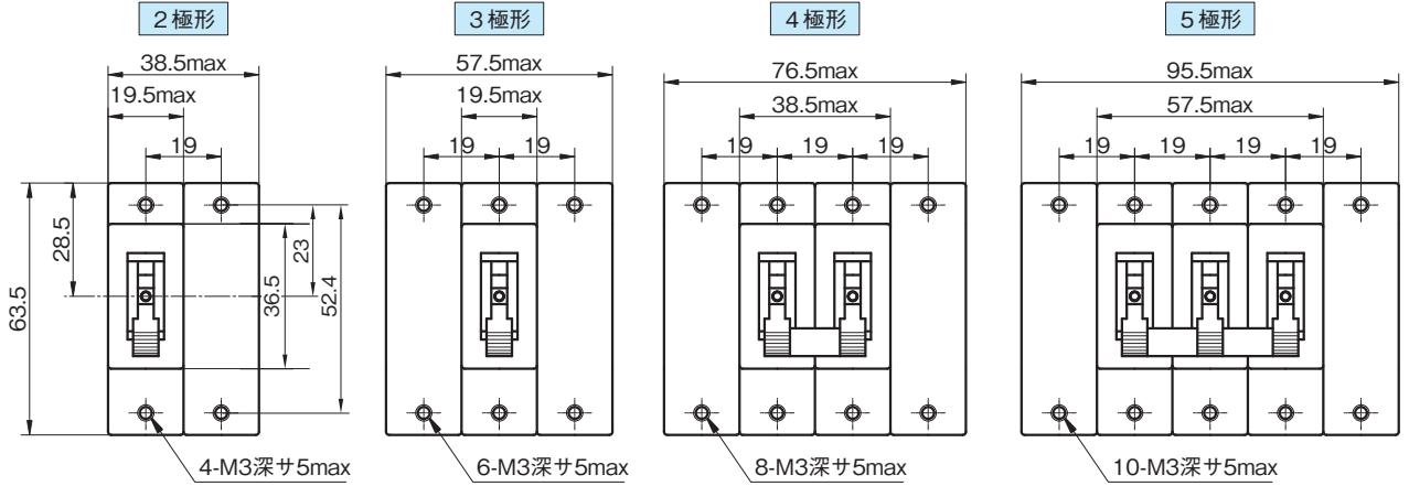
取付穴加工図 (公差±0.1)
