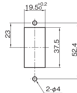
取付穴加工図 (公差±0.1)
