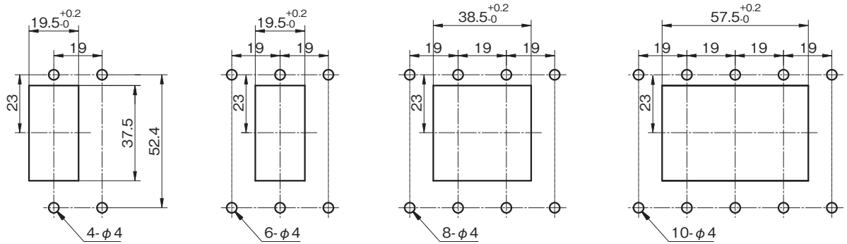
取付穴加工図 (公差±0.1)
