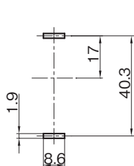
基板穴加工図 (公差±0.1)
