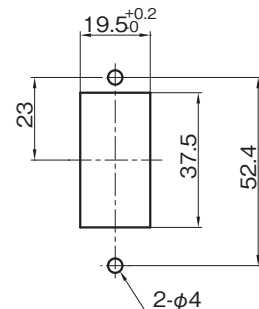
取付穴加工図 (公差±0.1)
