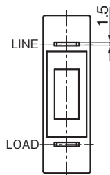
基板穴加工図 (公差±0.1)
