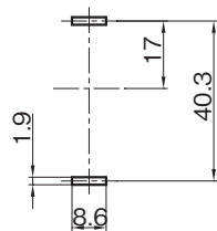
基板穴加工図 (公差±0.1)
