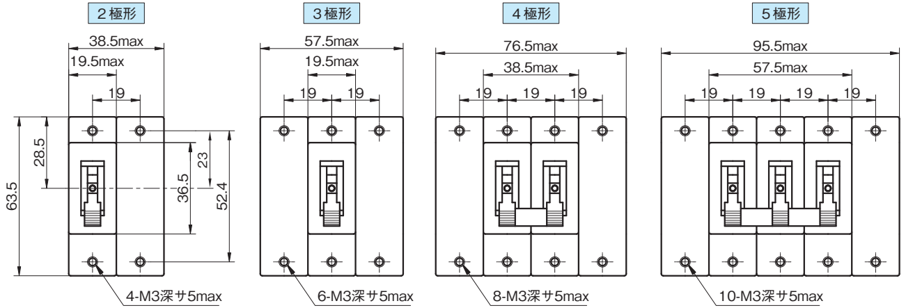
取付穴加工図 (公差±0.1)
